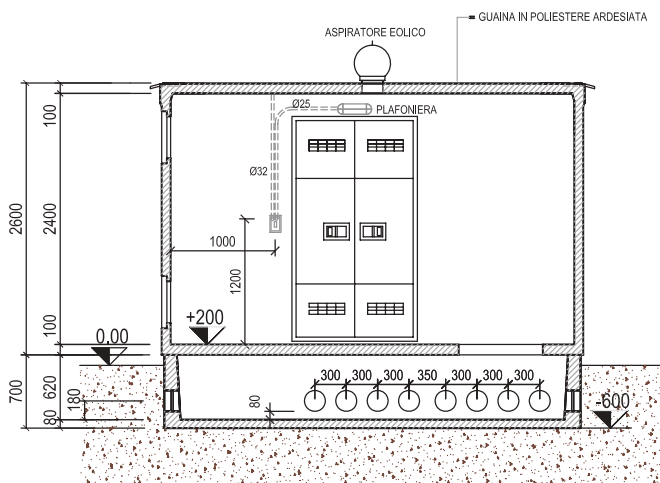
SEZIONE B-B
